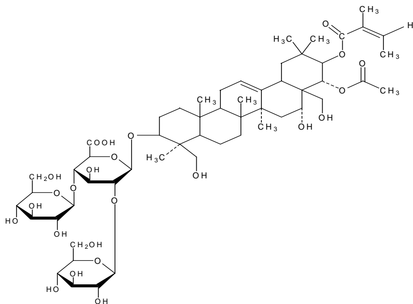
七叶皂苷 A 化学结构式
