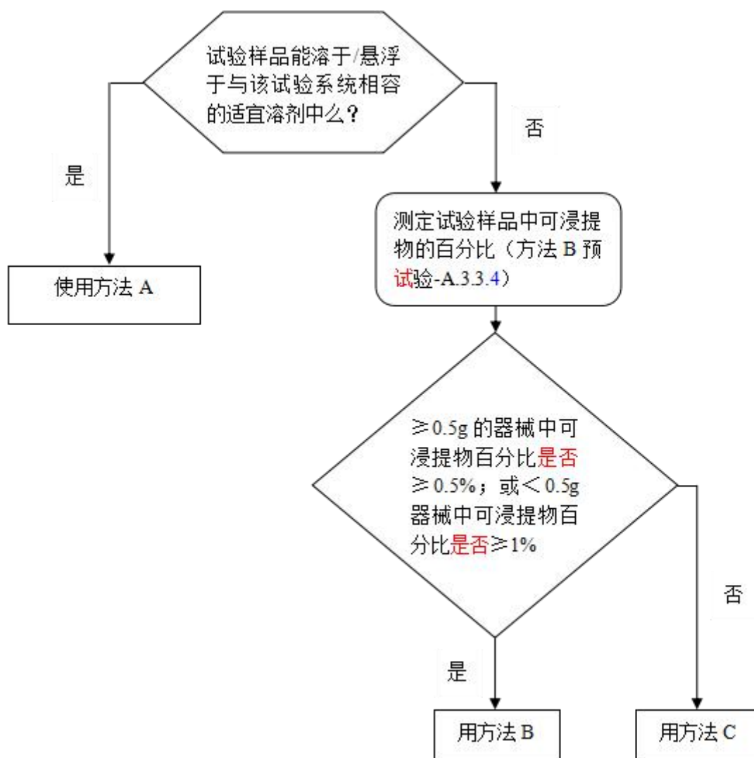
图 A.1 选择某一样品制备步骤的结构化方法
